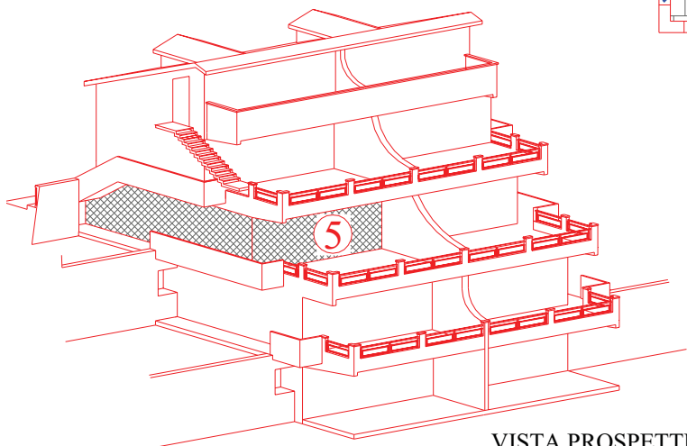
VISTA PROSPETTICA MODULO A3 - "SALINA"
